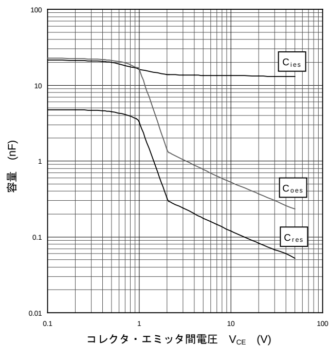
ゲート容量特性 (代表例)
