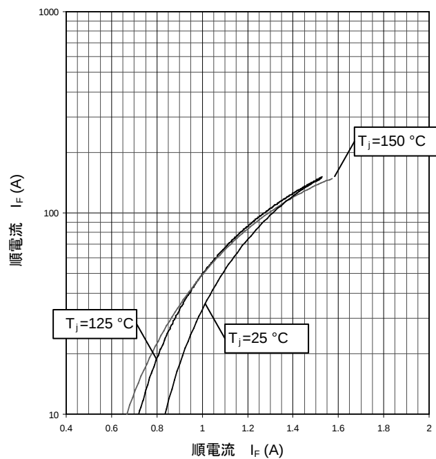
温度特性 (代表例)
