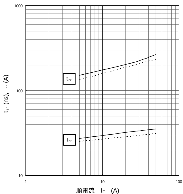
クランプダイオード逆回復特性 (代表例)
