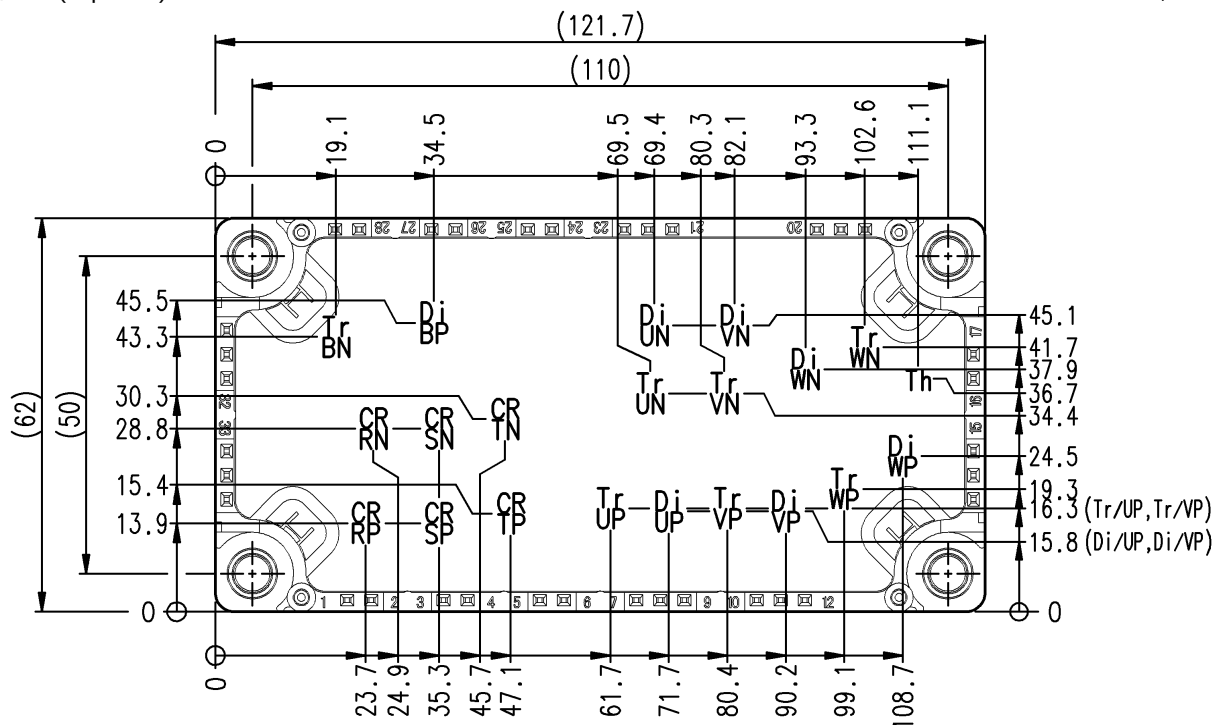
チップ配置図 (Top view)
