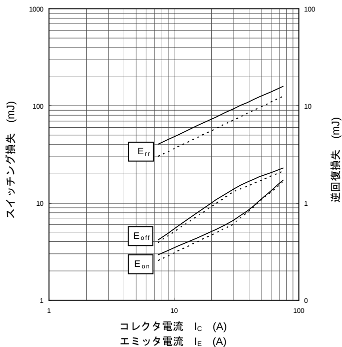
スイッチング損失特性 (代表例)
