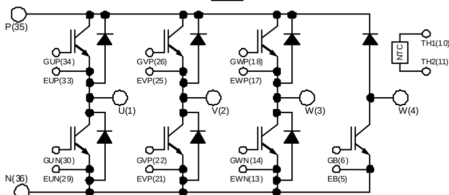
接続図
