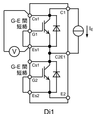
V_{EC} 試験回路
