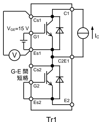
V_{CEsat} 試験回路
