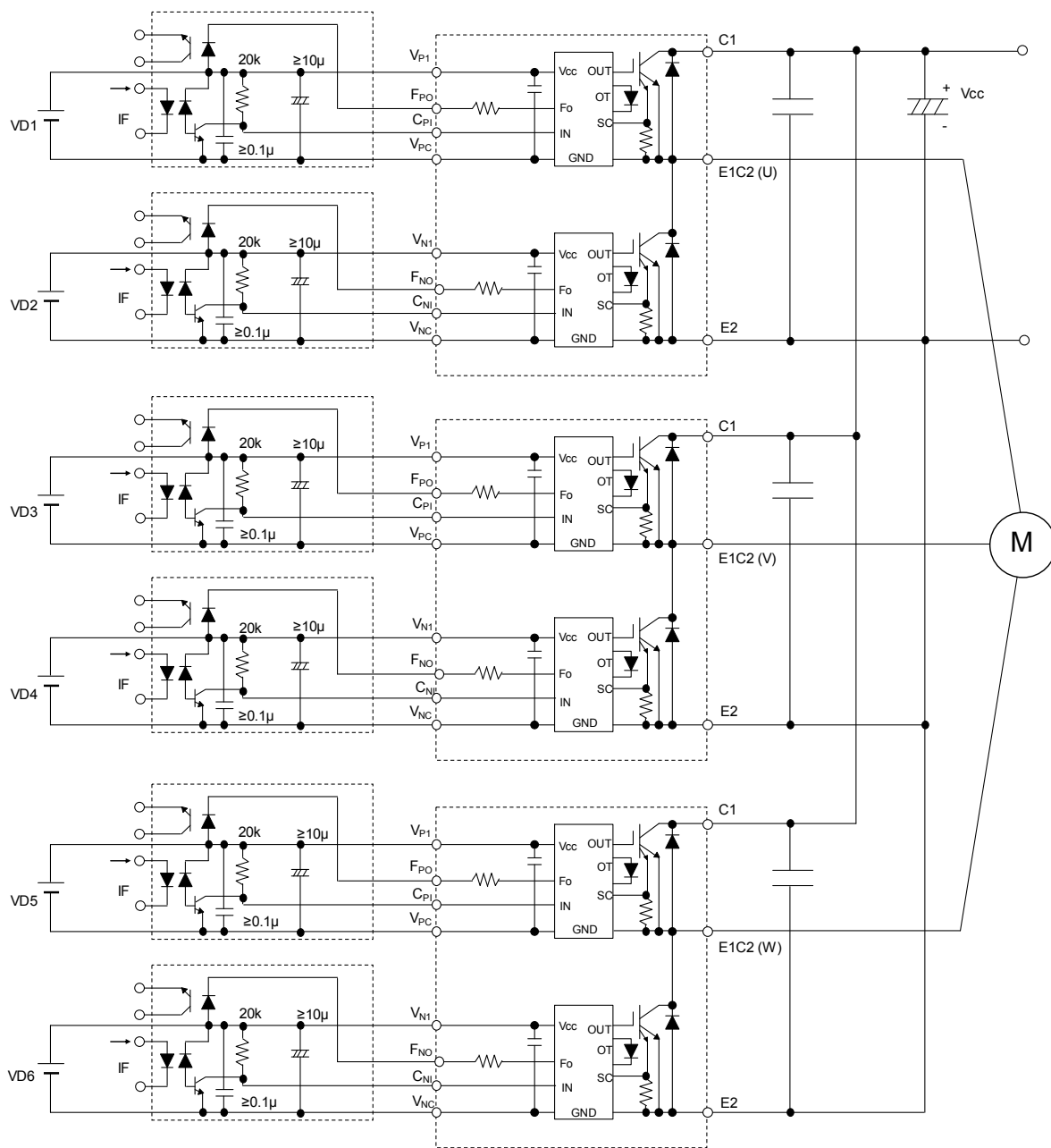
図 8. 応用回路例
