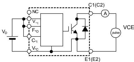
図 5. I_{CES} 試験
