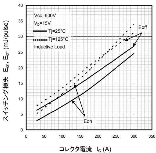
スイッチング損失特性 (代表例)
