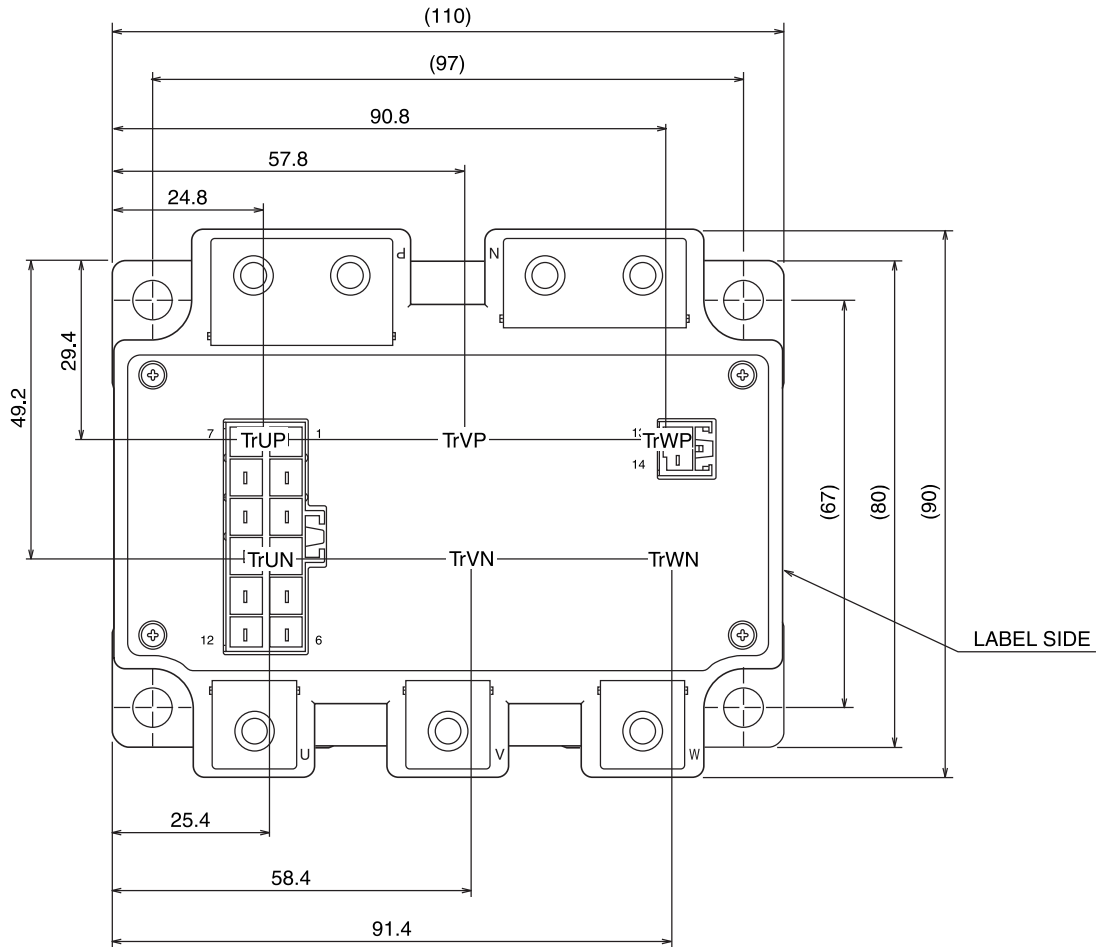
チップレイアウト図
