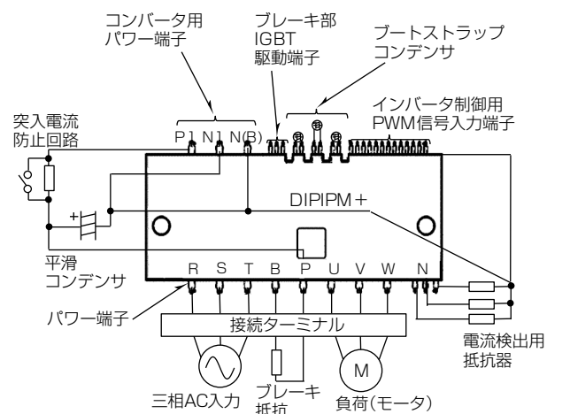
(b) DIPIPM+使用時の配線イメージ
