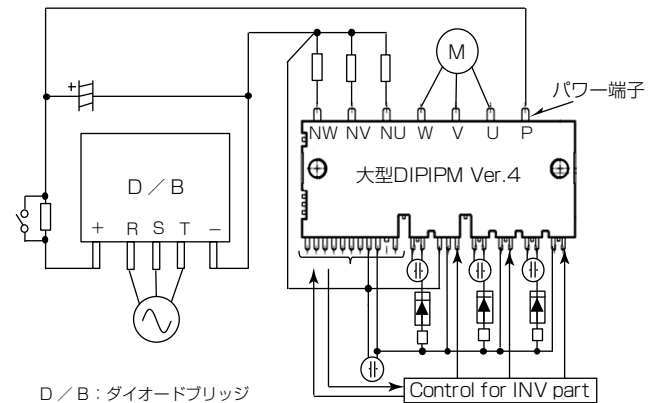
(a) 大型DIPIPM Ver.4使用時の配線イメージ
