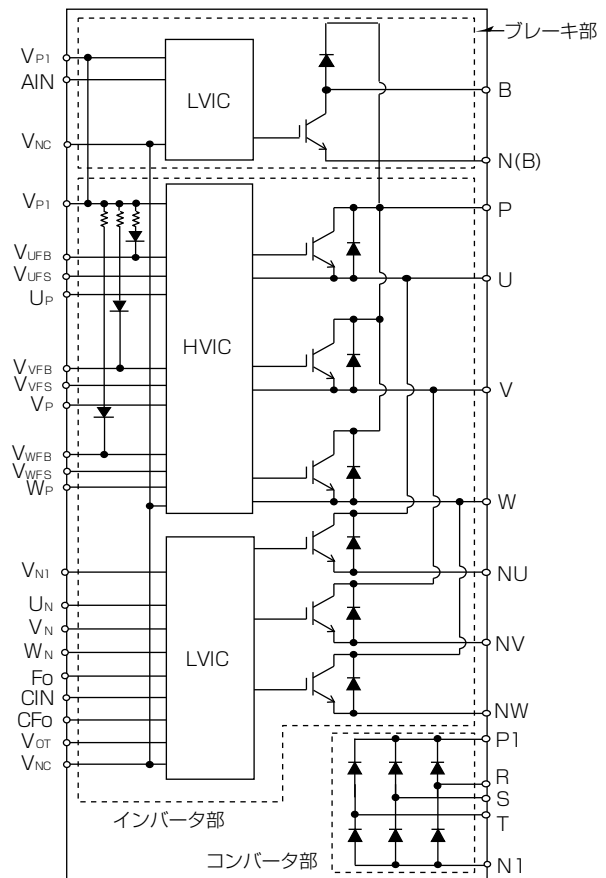
図1. 内部回路図
