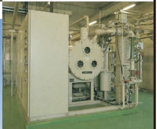
▼ オゾン発生装置 (弊社製)
